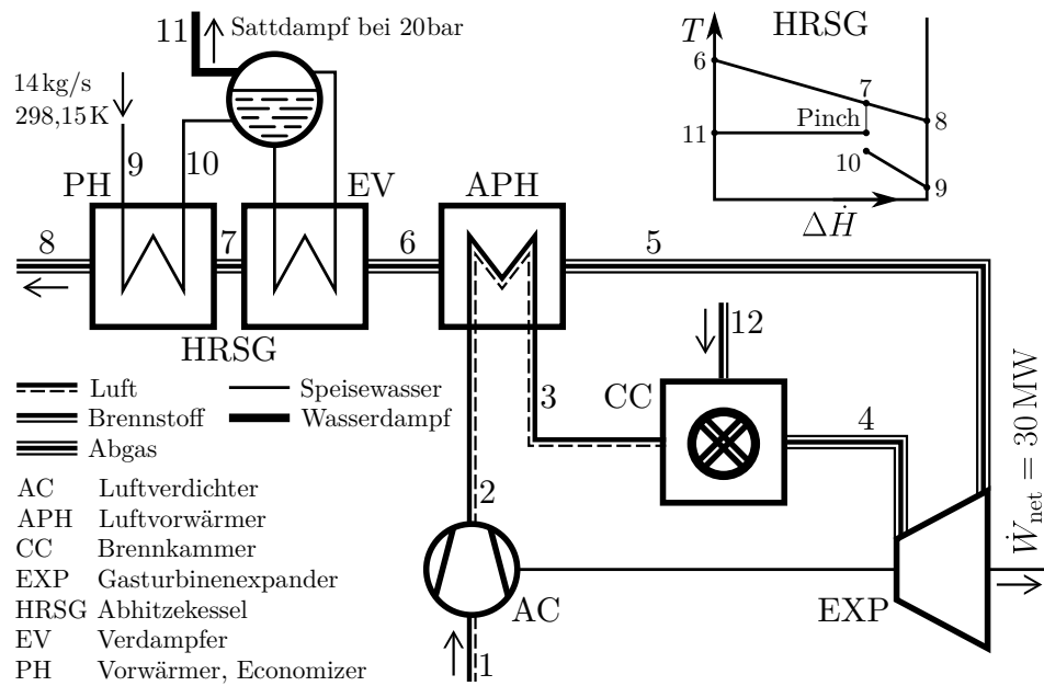
Abb. 2: Fließbild CGAM-Prozess
